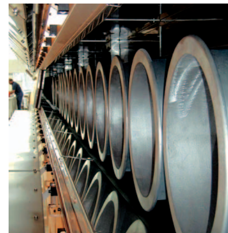
LCM 型盐浴硫化装置 / Salt bath type LCM
